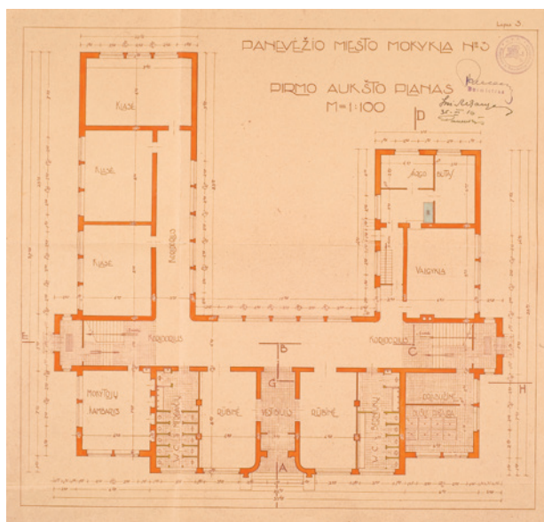
8 paveikslas. Buvusios 3-iosios pradinės mokyklos pirmo aukšto planas (LCVA, F. 1622, ap. 4, b. 476, l. 3)
